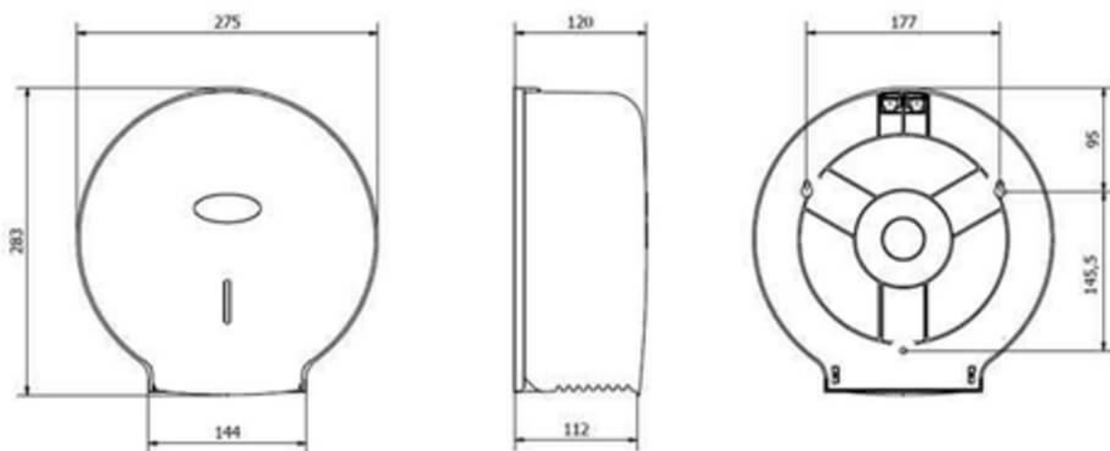
Podajnik Jofel AE57600
