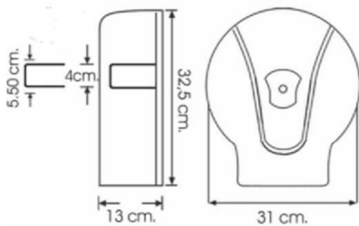
Schemat Podajnika
