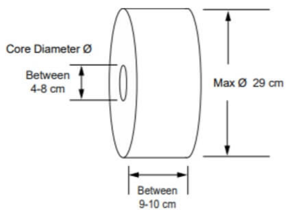
Rolka Papieru
